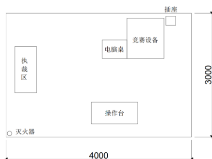
图 五-1 工业机器人系统操作员 S 竞赛工位布局示意图——职工组
